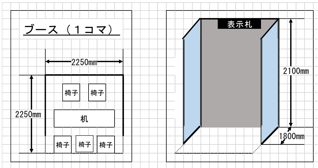
ブース設営図
